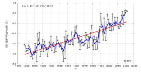
細線（黒）：各年の平均気温の基準値からの偏差、太線（青）：偏差の5年移動平均値、直線（赤）：長期変化傾向。基準値は1991～2020年の30年平均値。
